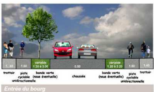
SEQUENCE CC' - Croix de Bel - Rés. Armand Drouart - 1/150
